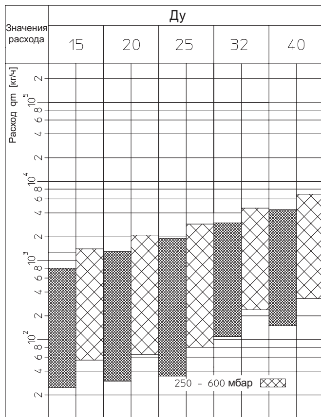
Значения расхода регулятора перепада давления „Hucoson DTZ“ при перепаде давления в стояке 50–300 мбар или 250–600 мбар и ограничение расхода на регулирующем вентиле „Hucoson VTZ“.
