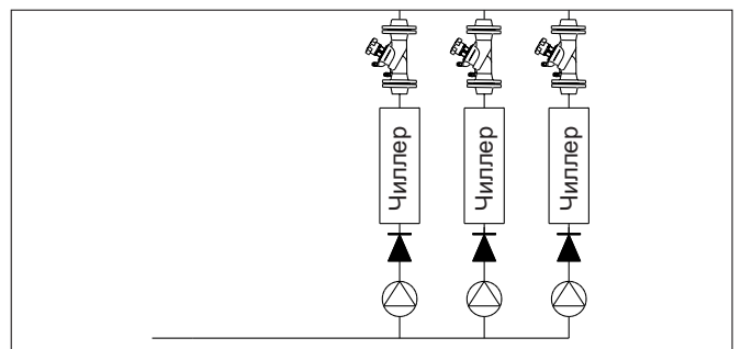
Пример: Система охлаждения с фланцевыми регулирующими вентилями.
