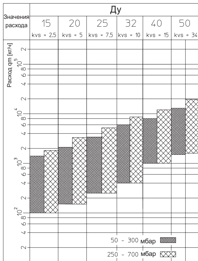
Значения расхода регулятора перепада давления „Нусоcon DTR“ при перепаде давления в стояке 50–300 мбар или 250–700 мбар.
