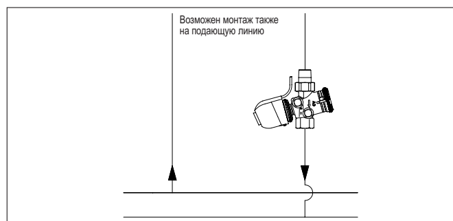
Пример: Регулирование расхода с помощью вентиля „Сосон QTZ“.
